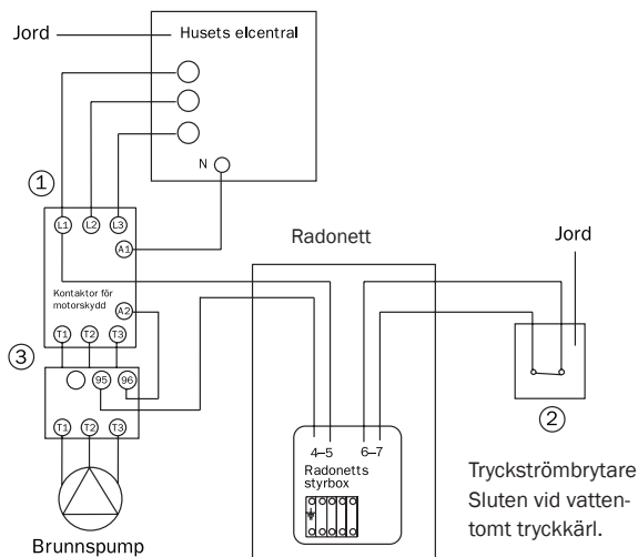
B Normal installation med Radonett utan filteranläggning
